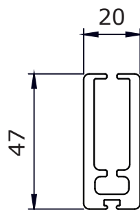
Barre de charge apparente aluminium (AR/BL/NR/GR)
