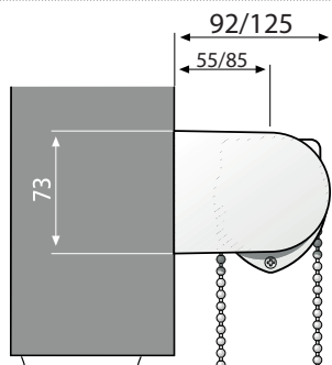
Supports décoratifs Déco - Gran Déco (AR/BL/NR/GR)
